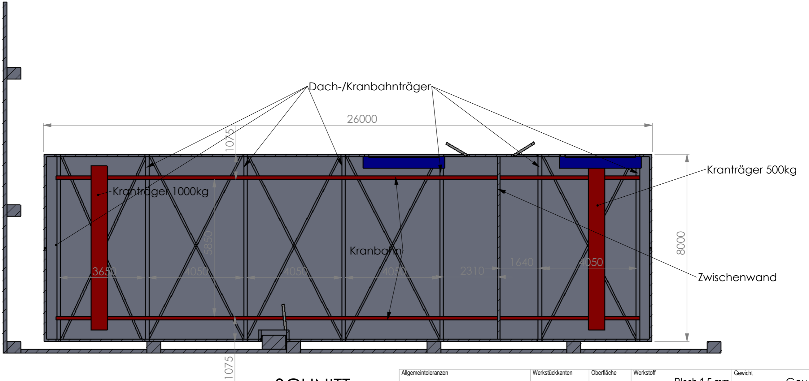
SCHNITT A-A MAßSTAB 1 : 100
