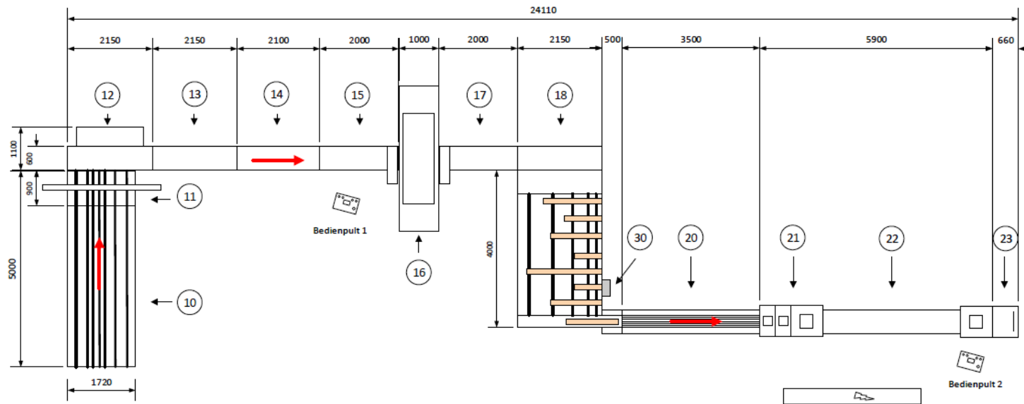
Layout SMB – 05
