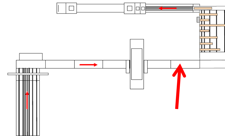
Layout SMB - 07
