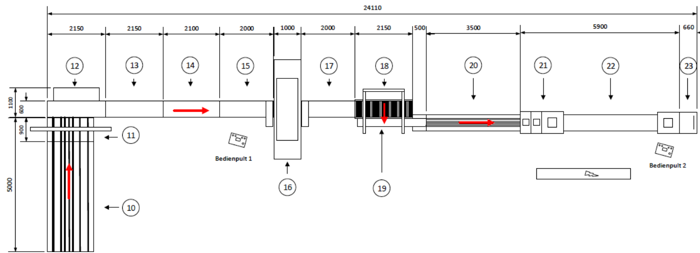
Layout SMB - 05
