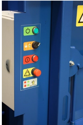
PLC-Steuerung mit automatischem Presszyklus
